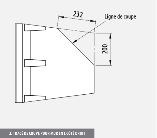
2. TRACÉ DE COUPE POUR MUR EN L CÔTÉ DROIT
