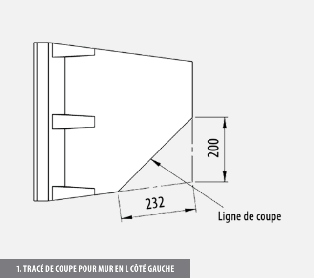
1. TRACÉ DE COUPE POUR MUR EN L CÔTÉ GAUCHE
