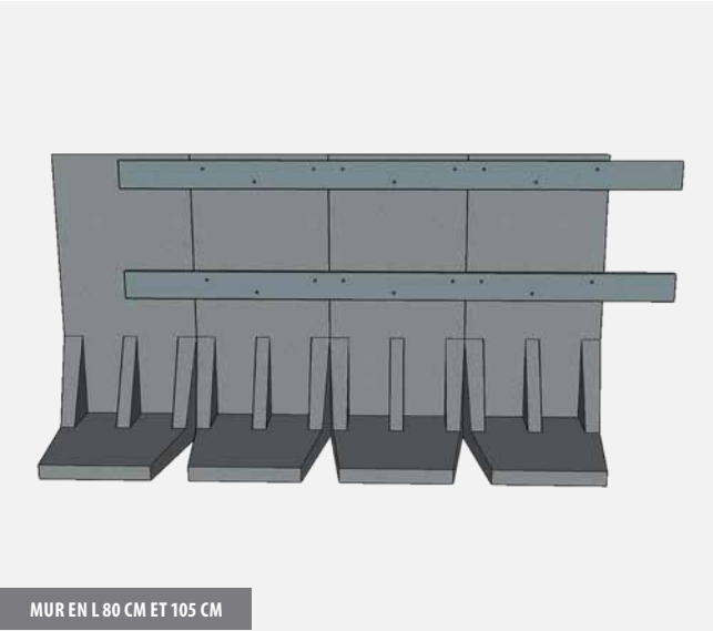
MUR EN L 80 CM ET 105 CM
